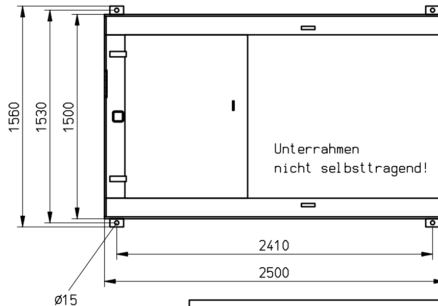
Maßblatt ELS 4-16-18
